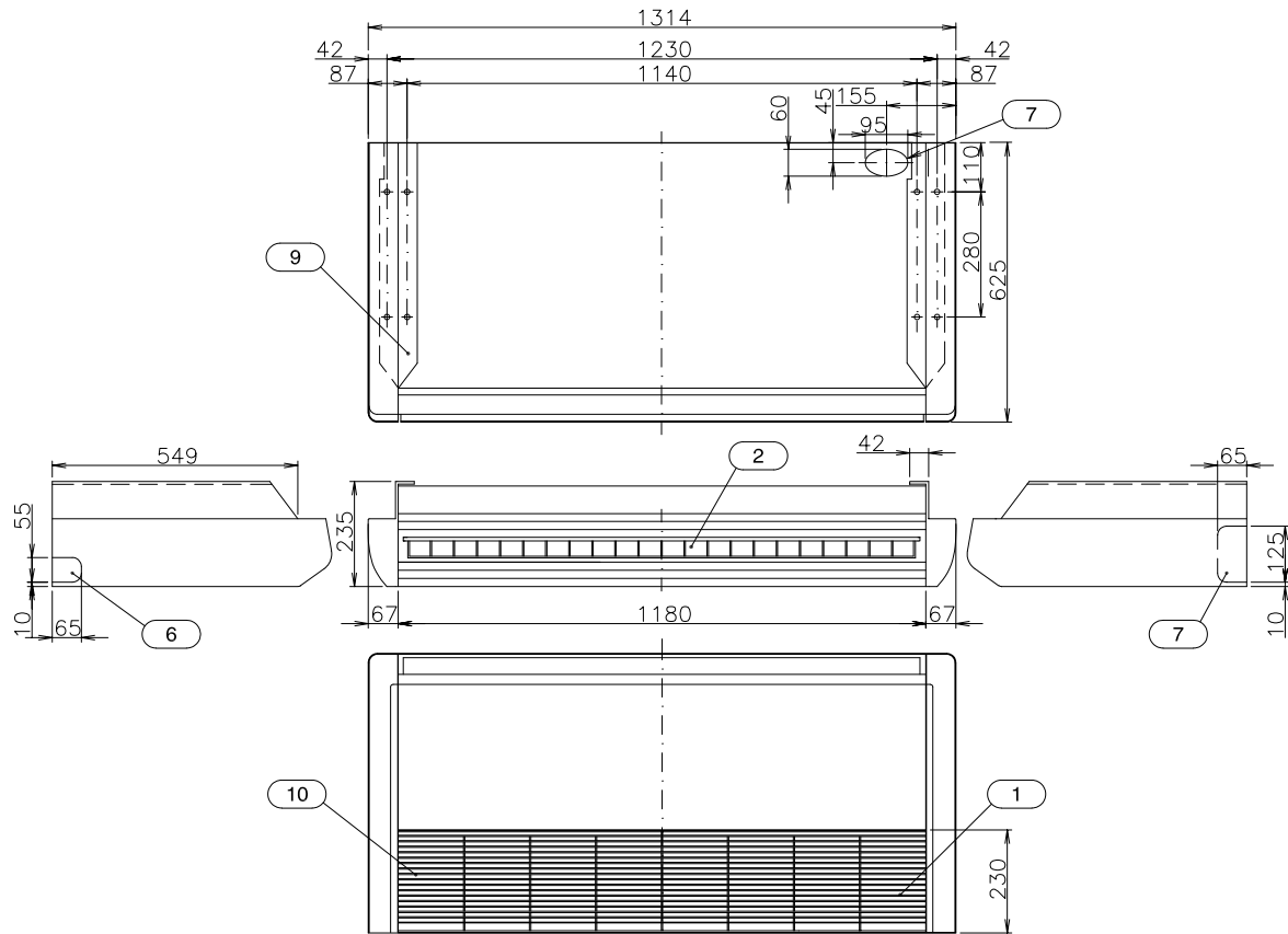
Anordnung Rohranschluss
