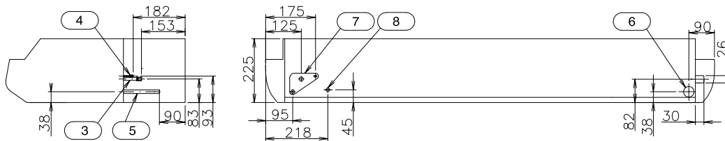
Platzbedarf
