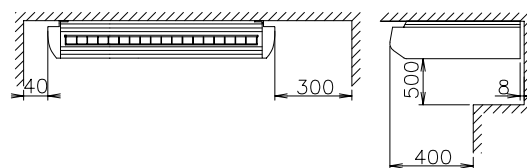
Platzbedarf
