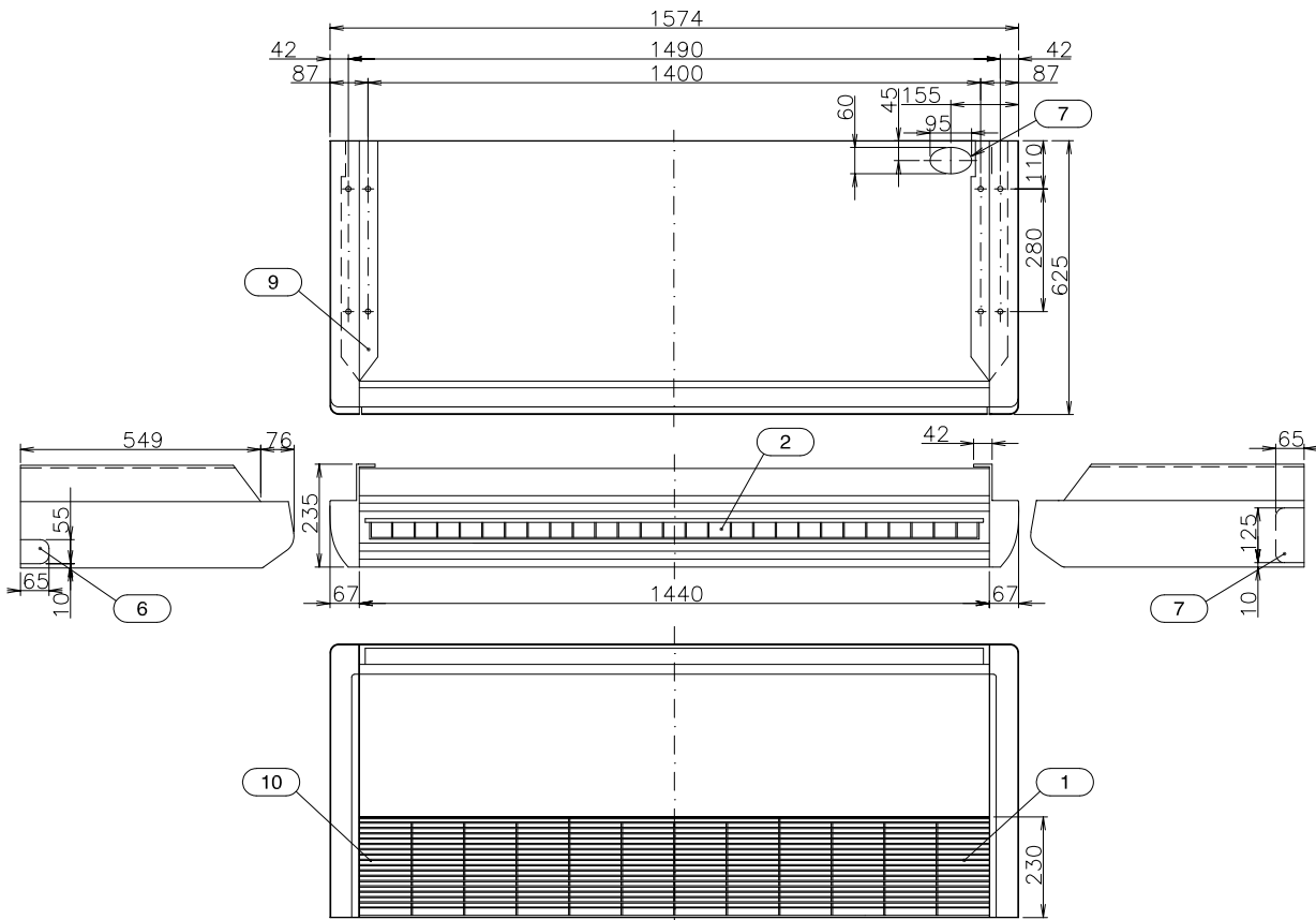
Anordnung Rohranschluss
