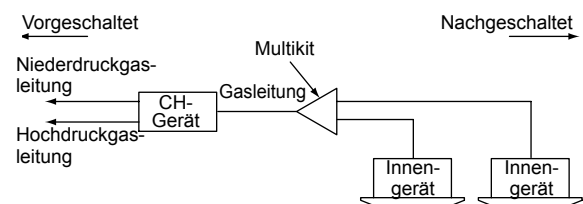
Bedingung bei Verlegung der Leitungen
